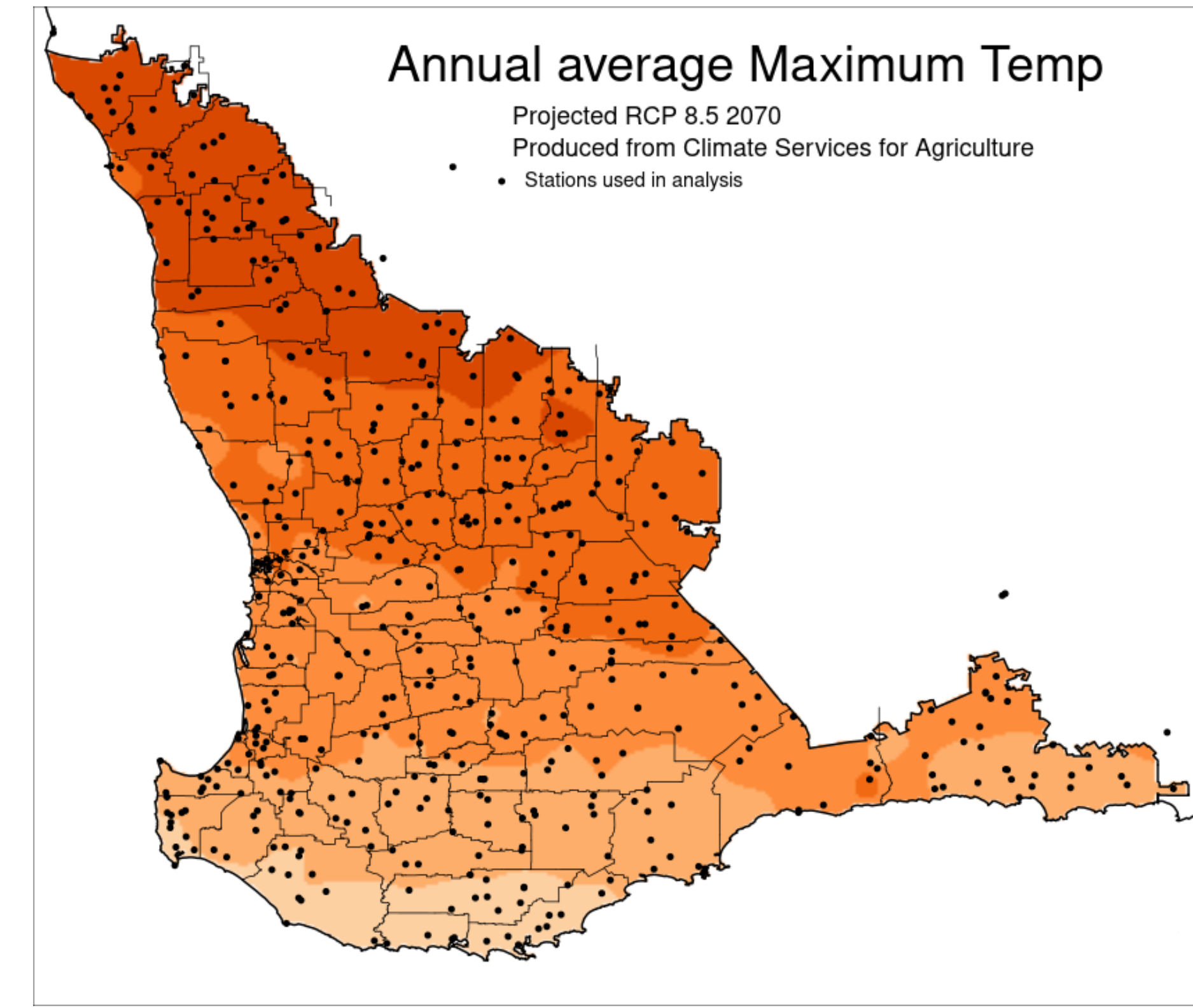
RCP 8.5 2070
