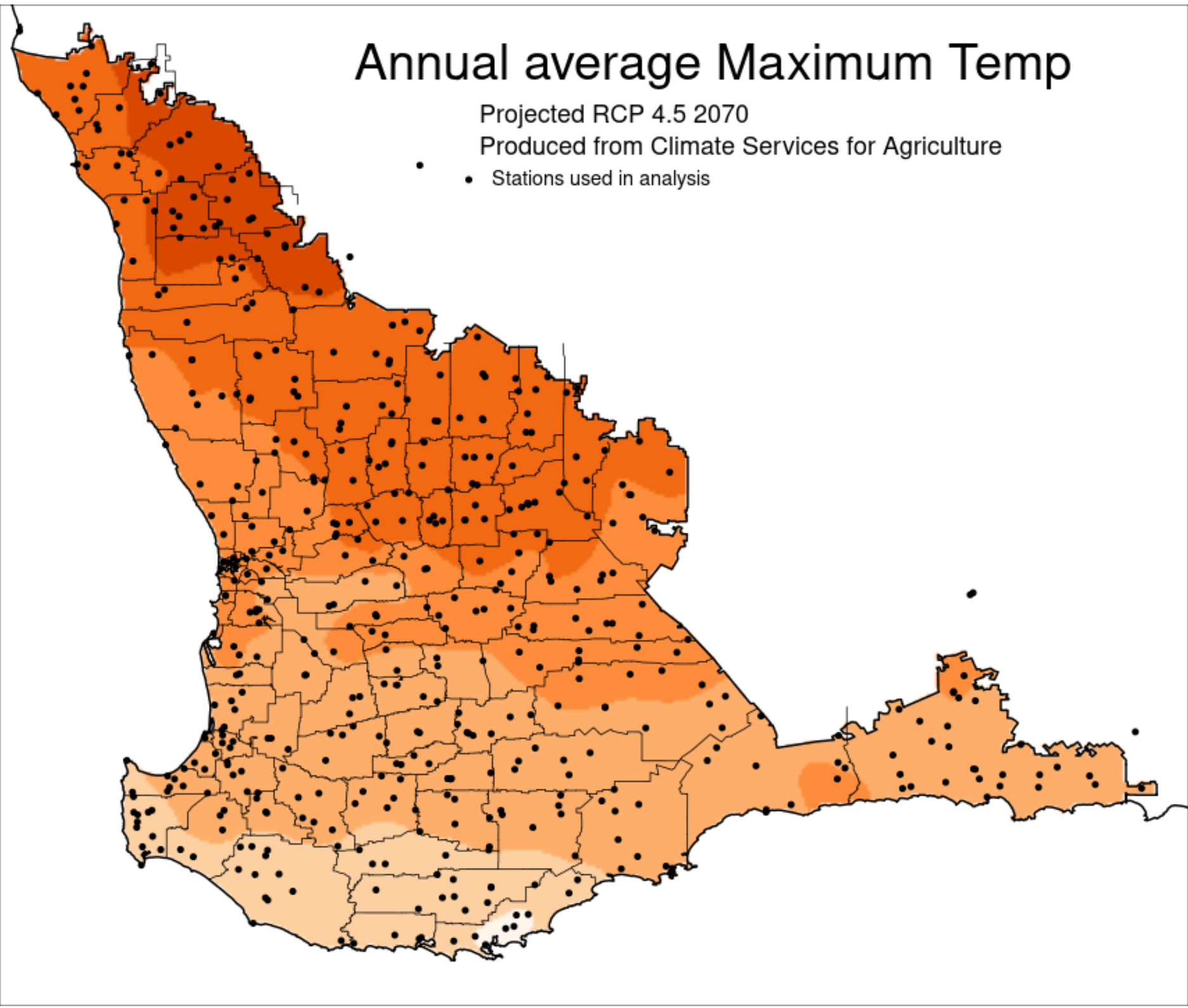
RCP 4.5 2070
